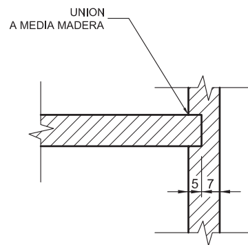
DETALLE 2 - TIPICO - Esc: 1/2
