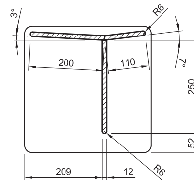
MODULO EDUCADORA - CORTE A -
