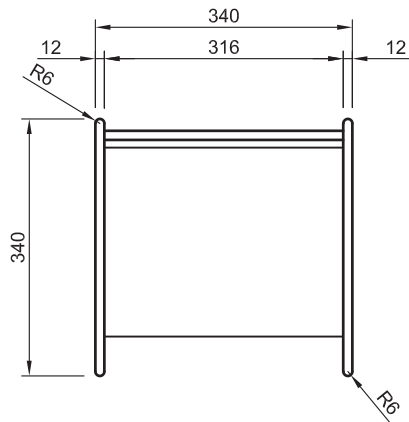
MODULO EDUCADORA - ELEVACION -
